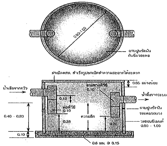
ปอดักไขมันแบบวงขอบซีเมนต์สำหรับบ้านพักอาศัย
