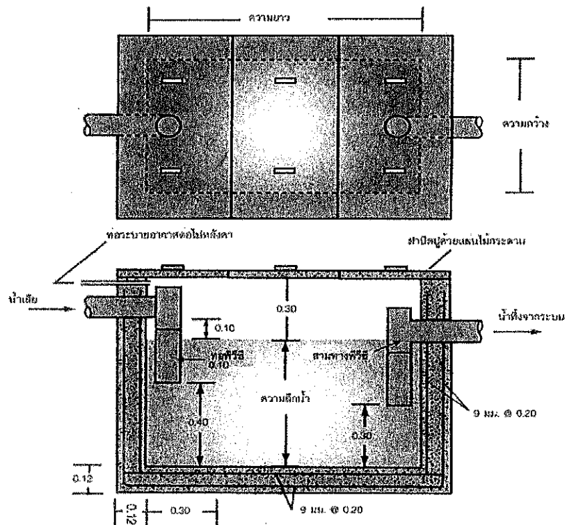
ปอดักไขมันแบบสร้างในที่สำหรับอาคารขนาดใหญ่
